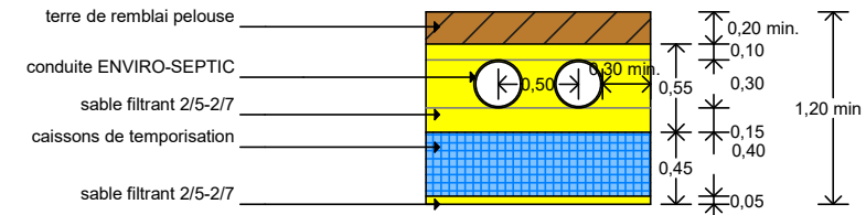
COUPE TRANSVERSALE
