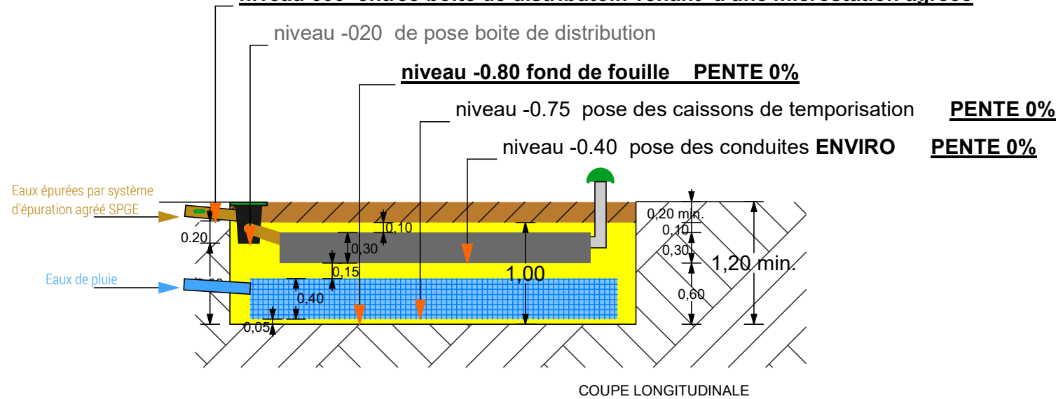
COUPE LONGITUDINALE
