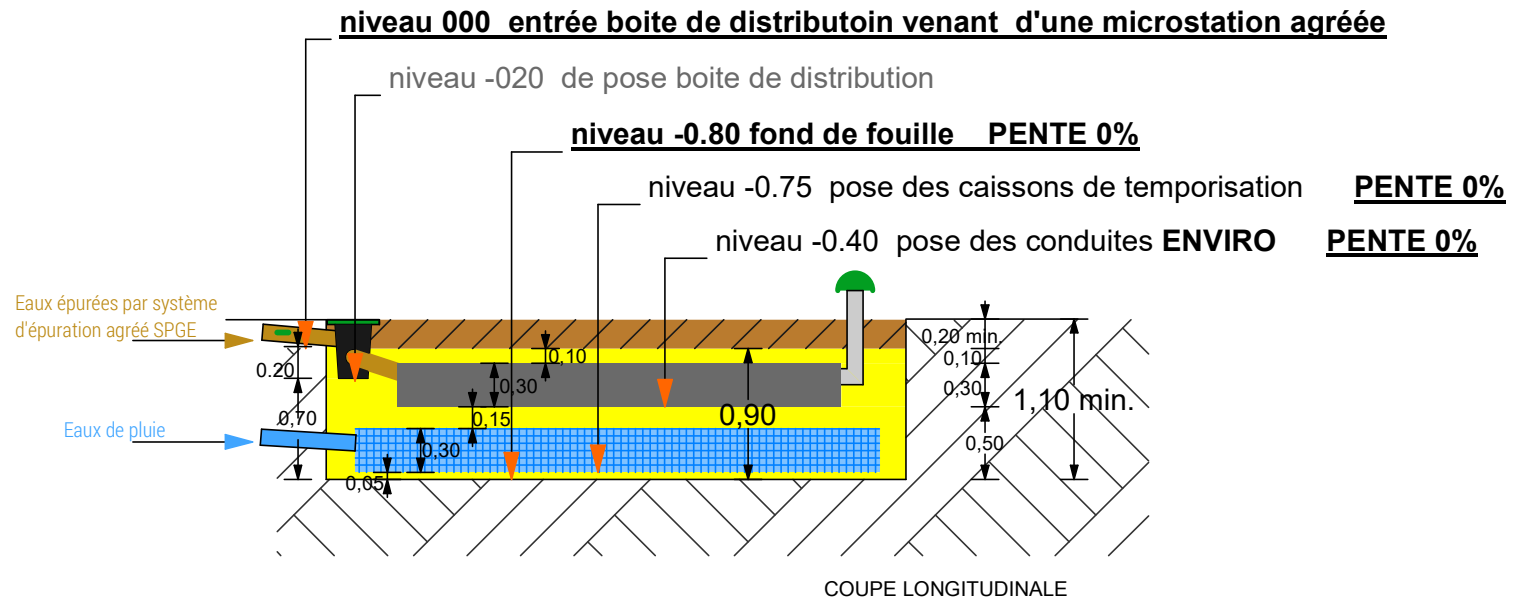
COUPE LONGITUDINALE
