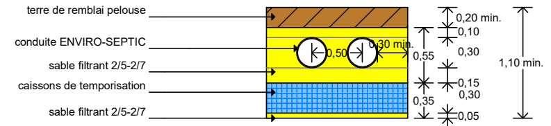
COUPE TRANSVERSALE
