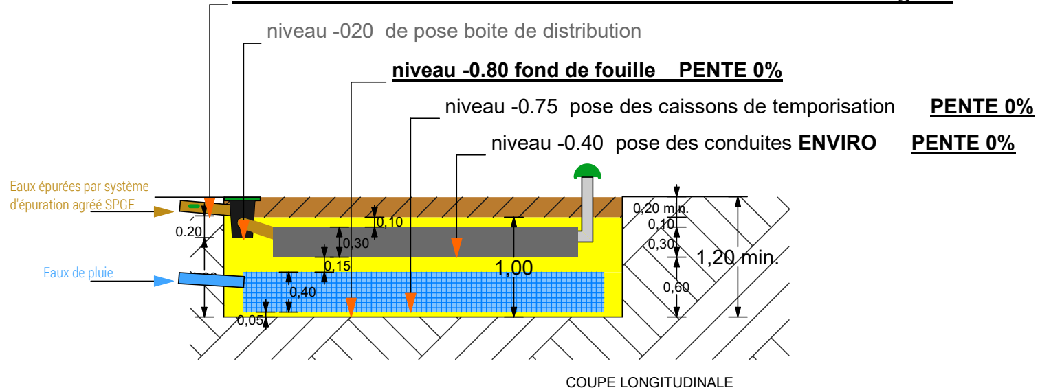
COUPE LONGITUDINALE
