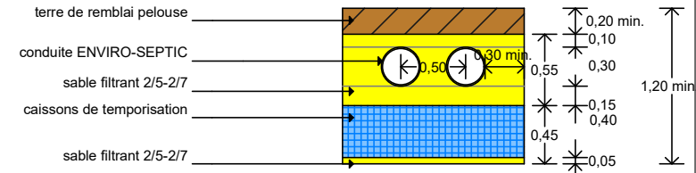
COUPE TRANSVERSALE
