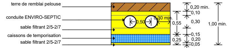
COUPE TRANSVERSALE
