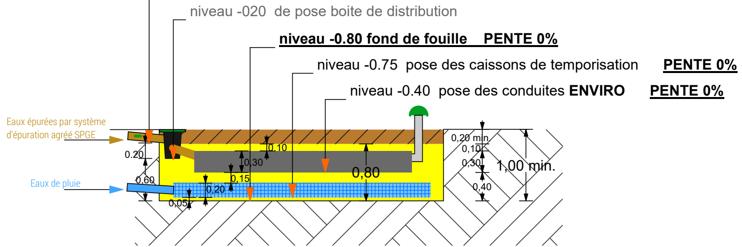
COUPE LONGITUDINALE
